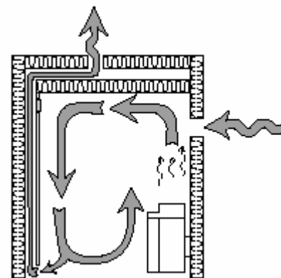
Пример правильной вентиляции сауны. Более подробные сведения о вентиляции приводятся на листе 25.
