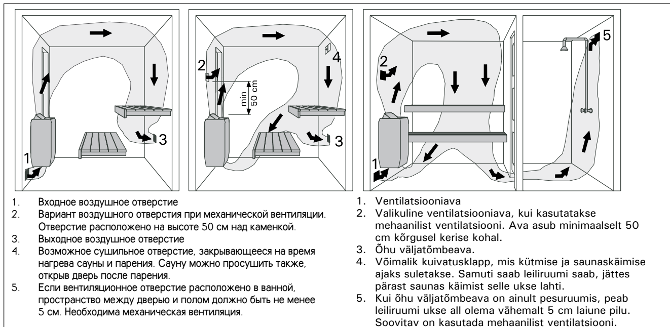
Рис. 2 Вентиляция в сауне Joonis 2. Leiliruumi ventilatsioon
