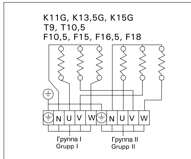
Рис. 5. Схема электроподключений каменки, установленной в качестве групповой Joonis 5. Kerise elektriühendus kahes grupis
