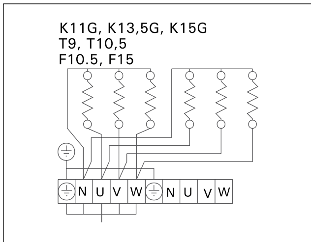
Рис. 4. Электромонтаж каменки Joonis 4. Kerise elektriühendus
