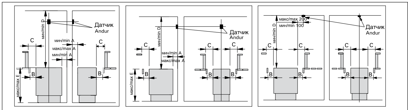
Рис. 3. Безопасные расстояния каменки. Вним.! Если значение E больше E макс., то И мин. = C мин. Joonis 3. Ohutuskaugused kerisest. Märkus! Kui E on kõrgem kui E max, siis B min = C min.
