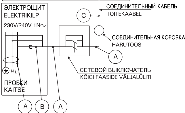
Подключение в 1-фазной сети, 230V~ Kerise 1-faasilised elektrühendused, 230V~
