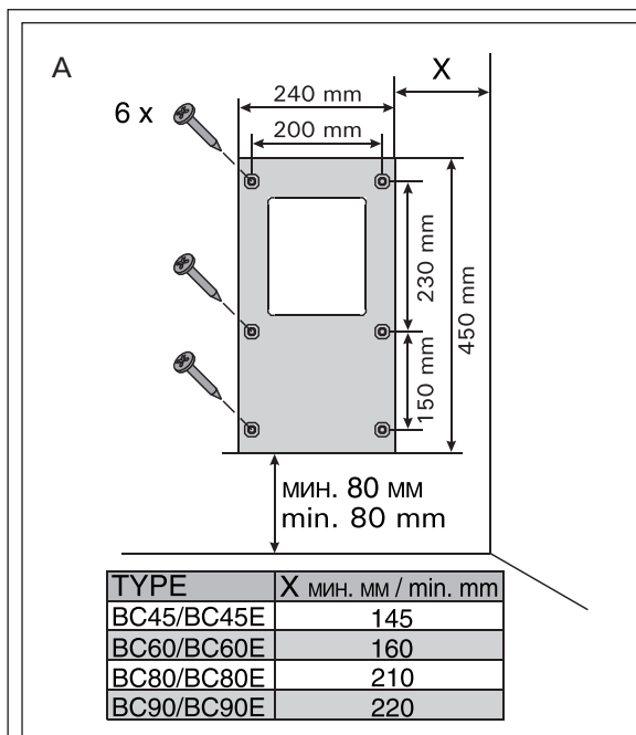
Рисунок 5. Расстояния безопасности Joonis 5. Kerise ohutuskaugused
