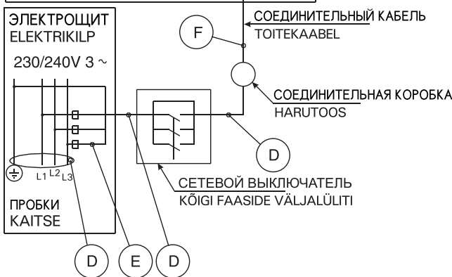
Подключение в 3-фазной сети, 230V 3~ Kerise 3-faasilised elektrühendused, 230V 3~
