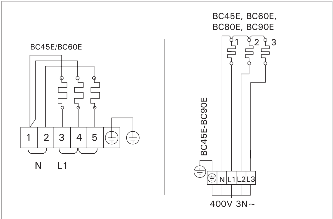
Рисунок 10а. Электромонтаж каменок мощностью 4,5 и 6,0 кВт для российского рынка
