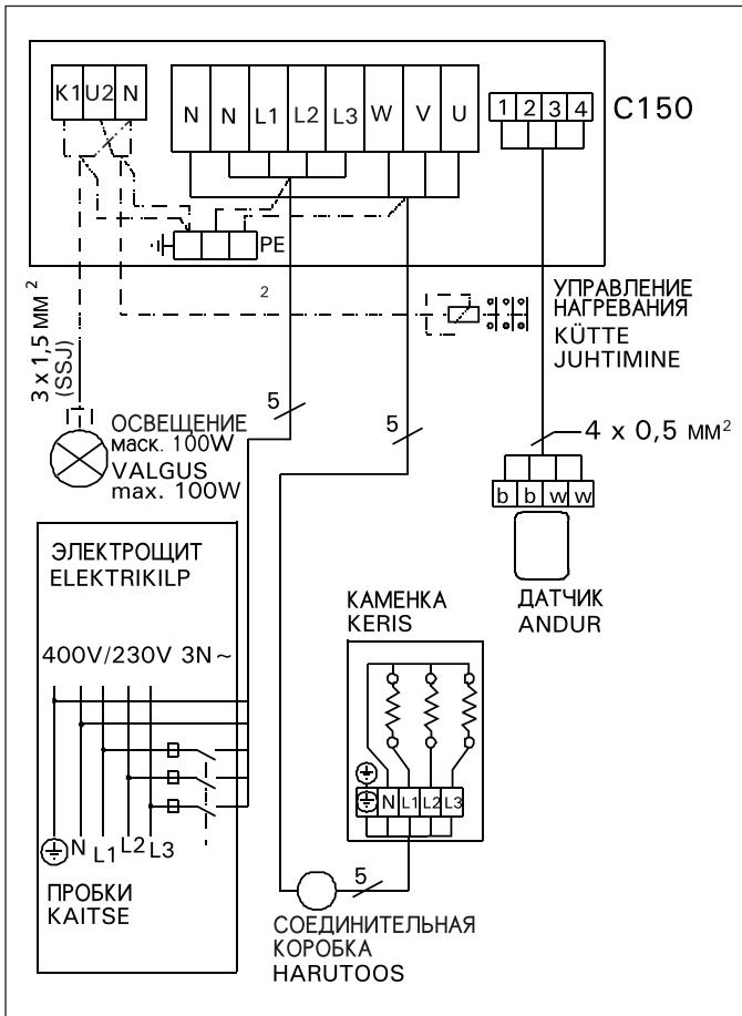
Рисунок 11б. Электромонтаж пульты управления C150 и каменки ВСЕ (подключение в 3-фазной сети)
