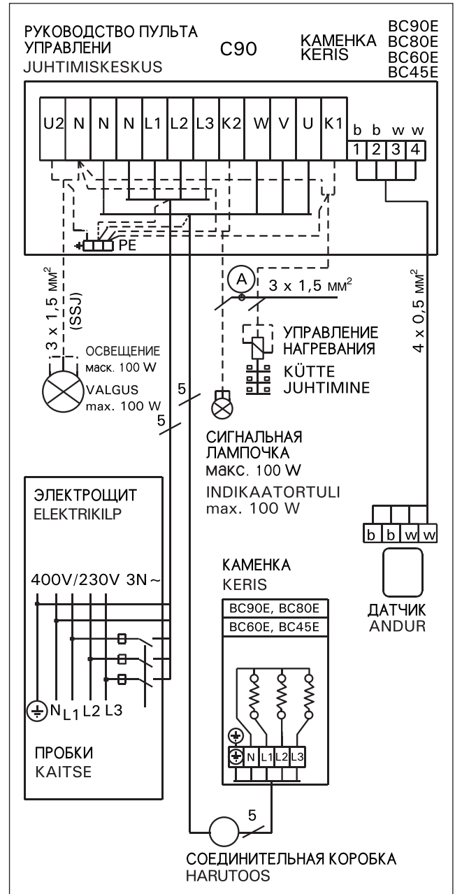
Рисунок 11в. Электромонтаж пульты управления C90 и каменки ВСЕ (подключение в 3-фазной сети)
