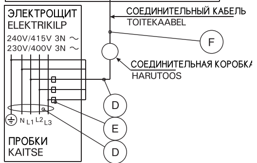
Подключение в 3-фазной сети, 400V 3N~ Kerise 3-faasilised elektrühendused, 400V 3N~
