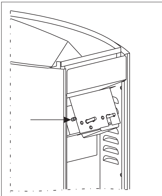
Рисунок 12. Кнопка возвращения предохранителя от перегрева
